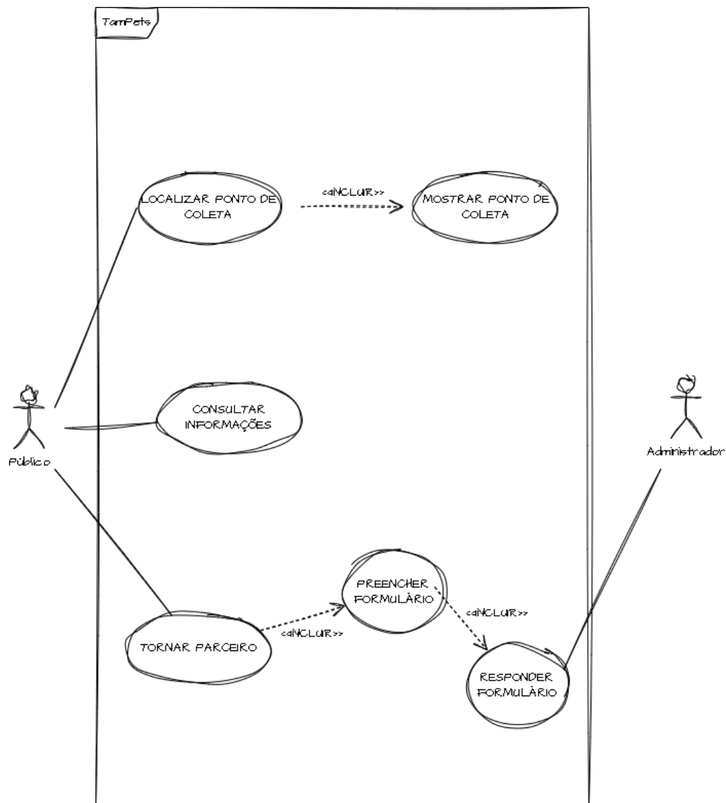
Figura 6 UML de caso de uso. Autor: Autoria Própria.
