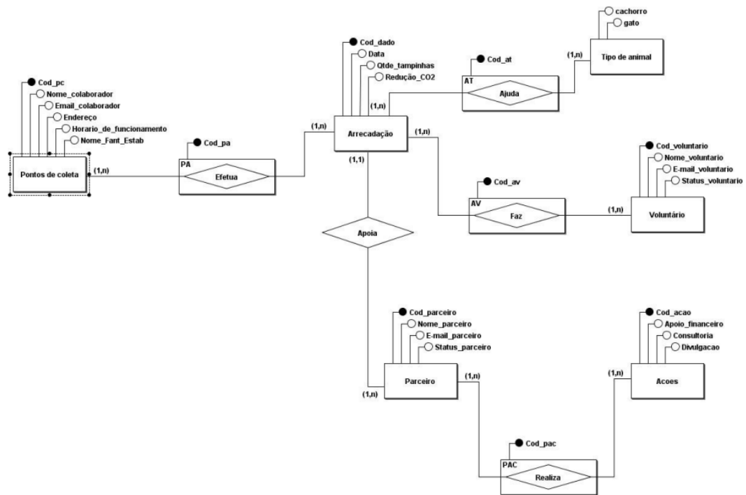
Figura 9 – Modelo Banco de Dados Conceitual. Autor: Autoria Própria.
